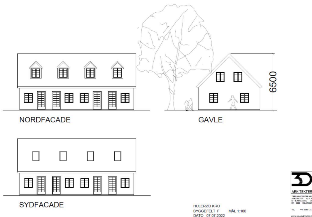
Illustration af mulig bygning til ferielejligheder på areal syd for Hulerødvej (bygning F).
